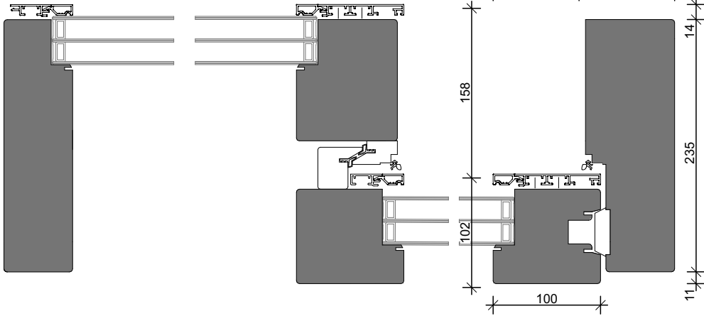
Jamb (1)
